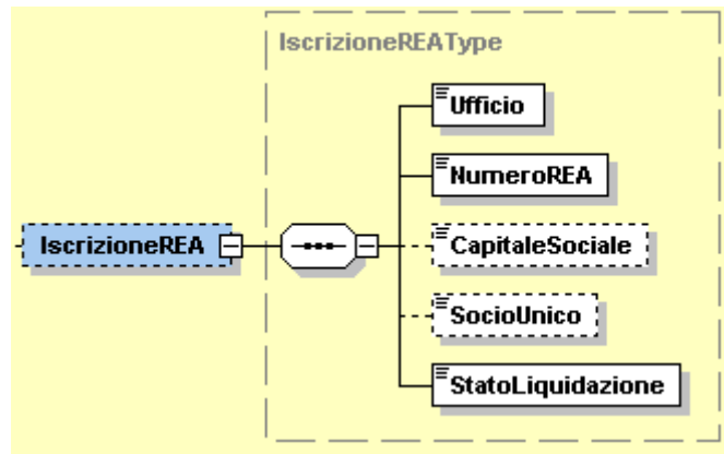
Figure 9: Element IscrizioneREA
